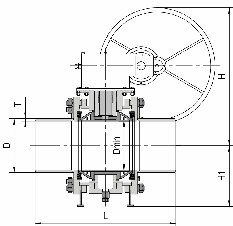
Схема монтажа крана шарового на фундаменте
