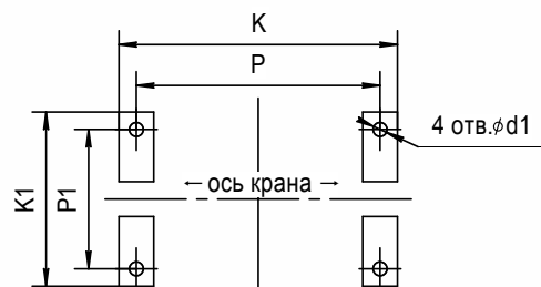
Схема монтажа крана шарового на фундаменте
