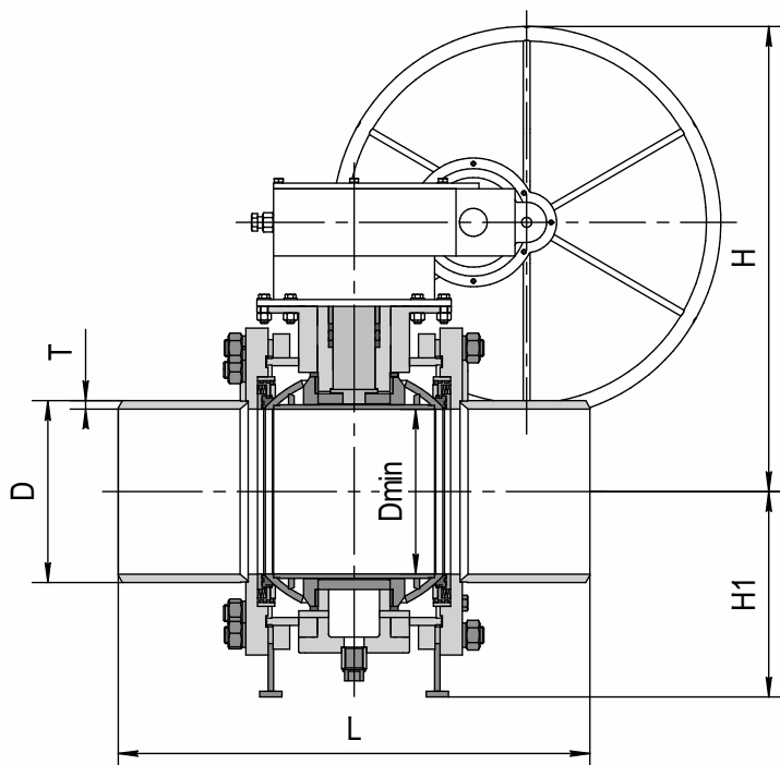
Схема монтажа крана шарового на фундаменте
