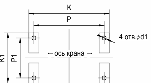
Схема монтажа крана шарового на фундаменте
